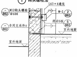
③ 滑动螺栓法
