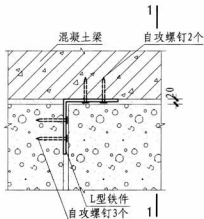
① 与混凝土结构连接
