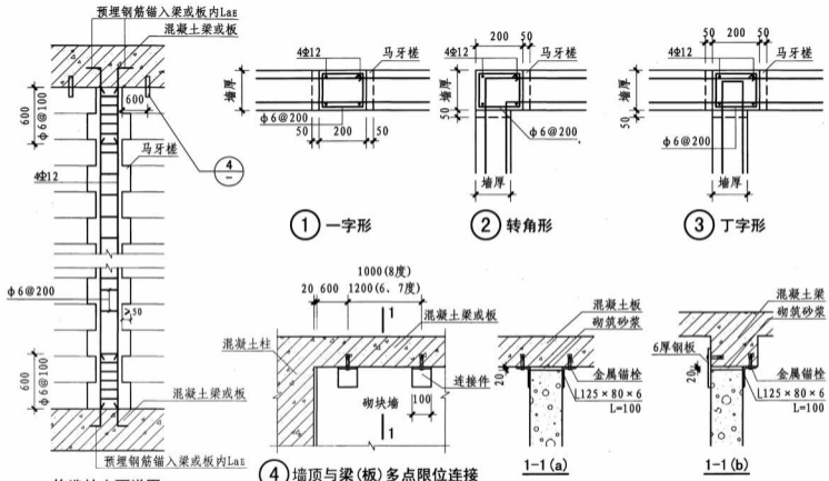
构造柱立面详图
