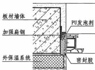
④ 塑料、铝合金门窗框，扁钢加强 ⑤ 塑料、铝合金门窗框，扁钢加强 ⑥ 塑料、铝合金门窗框，扁钢加强
