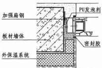
④ 塑料、铝合金门窗框，扁钢加强 ⑤ 塑料、铝合金门窗框，扁钢加强 ⑥ 塑料、铝合金门窗框，扁钢加强
